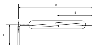
c) 剪脚&amp;弯脚
