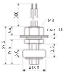
PLS-020 – Weltkleinster!
