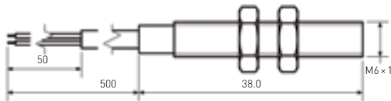
MS-226M
