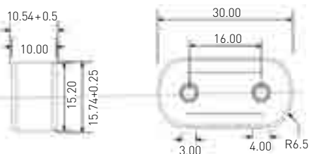
PFM-PP-Q001
