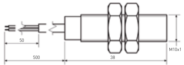
TS-2212M
