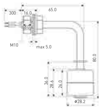
PLS-080
